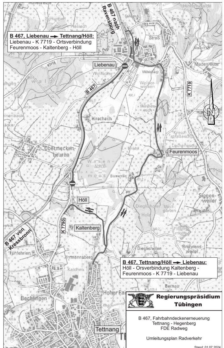
Umleitungsplan Radverkehr
