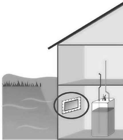
Variante 1: Aufstellraum gegen eindringendes Wasser sichern
